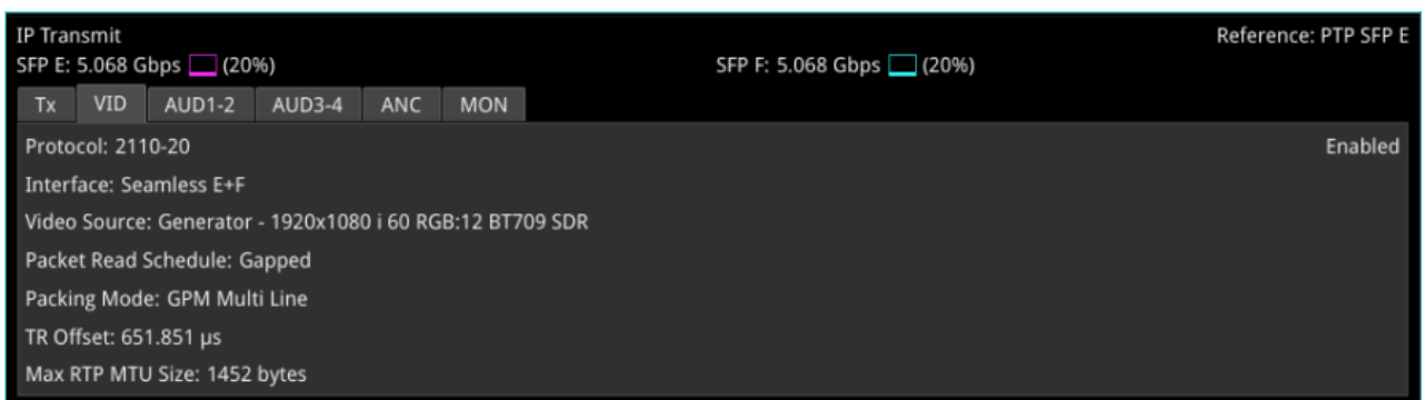
Figure 6-17: IP Transmit - VID Status Tab
